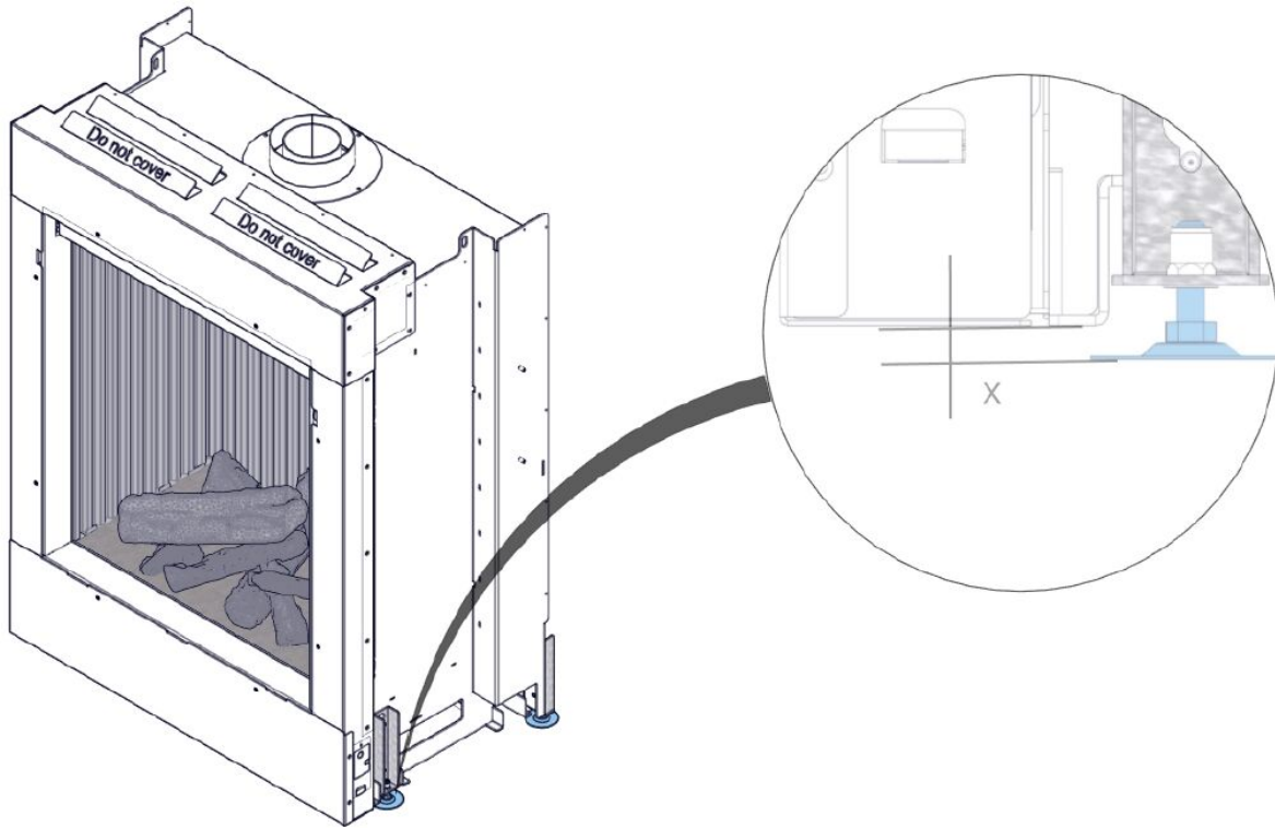
Abb. 4: Ausrichtung mittels Stellfüssen
